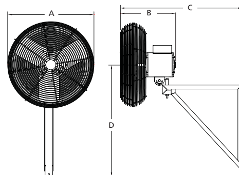
Figure 3 — Dimensions du 3PEG9A
