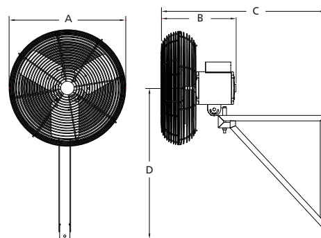
Figura 6 — Dimensiones de los Modelos 3PEH2A
