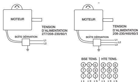
Figure 7 — Schéma de câblage typique
