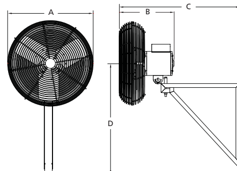
Figura 3 — Dimensiones 3PEG9A
